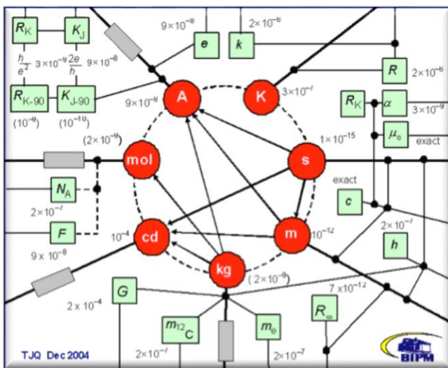
Figura 3 Relacionamento entre as unidades de base do SI e as constantes fundamentais [25].
