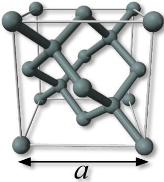
Figura 10 A célula unitária de silício tem um arranjo de empacotamento cúbico de faces centradas de 8 átomos com base. O volume da célula unitária é medido determinando o parâmetro de rede a , que é o comprimento de um dos lados do cubo [41].
