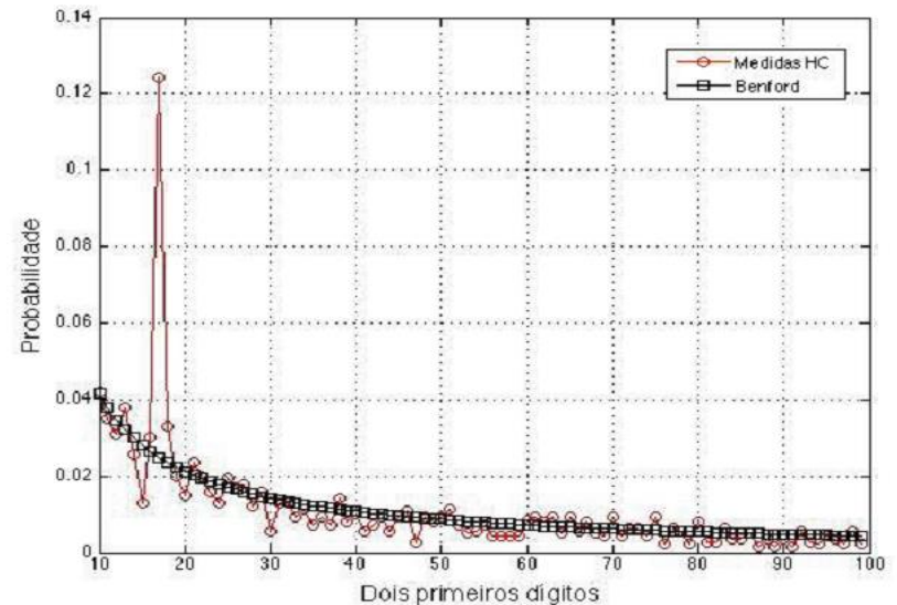
(b) Lei de Benford com os dois primeiros dígitos mais significativos
