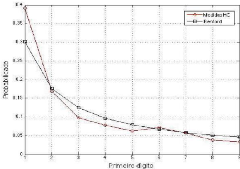
(a) Lei de Benford com o primeiro dígito mais significativo
