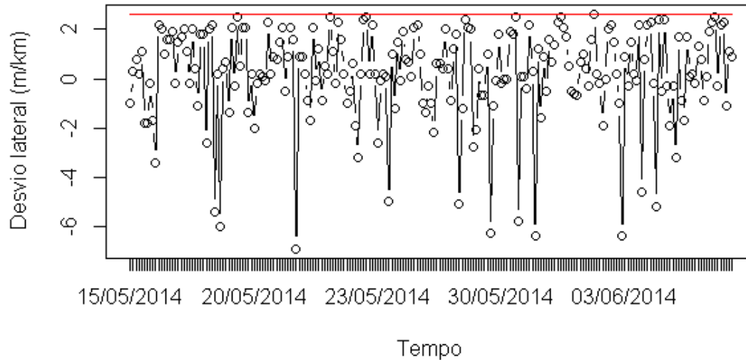
Medições de alinhamento de roda
